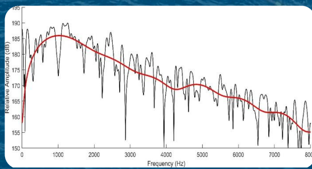
波形测试e-Boomer 300S @1000J
