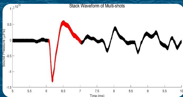
波形测试e-Boomer 300S @1000J
